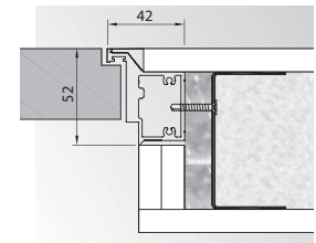
przeciw-przylga (otwierane do wewnątrz)
