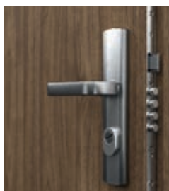
zamek listwowy wielobolcowy dostosowany pod dwie wkładki patentowe
